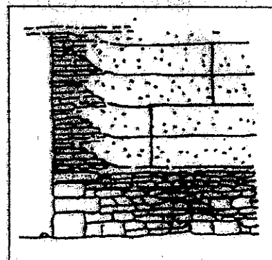
الشكل 17. معالجة الزوايا
