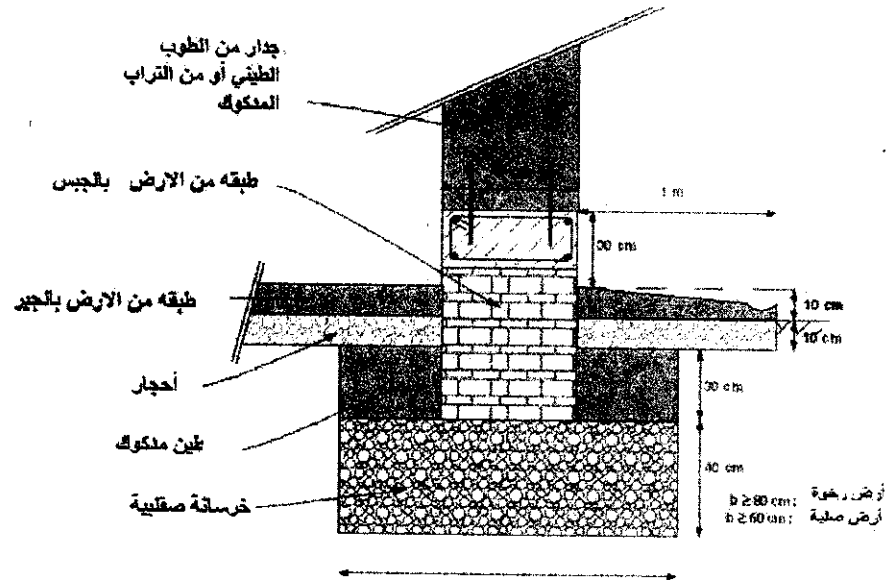
الشكل 50. أساس من خرسانة صقلوبية + ميطرات من الخرسانة المسلحة + أعمدة الربط جدار- ميطرة
