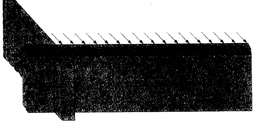
الشكل 9. تشققات أفقية الواصلة على مستوى الوصل بين الجدار والتسلسل الرابط
