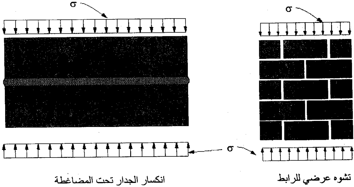
الشكل.22. انكسار البناء تحت مضاطعة بسيطة
