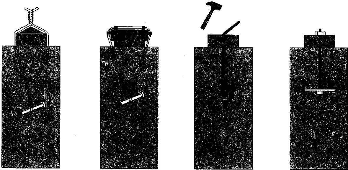
الشكل 41. أصناف الربط لميتره أفقية لجدار
