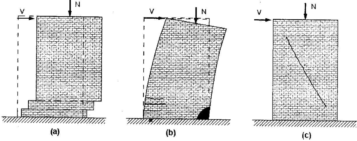
الشكل 24. طرق انكسار جدار من الطين معرض لحمولة في مسطحه
