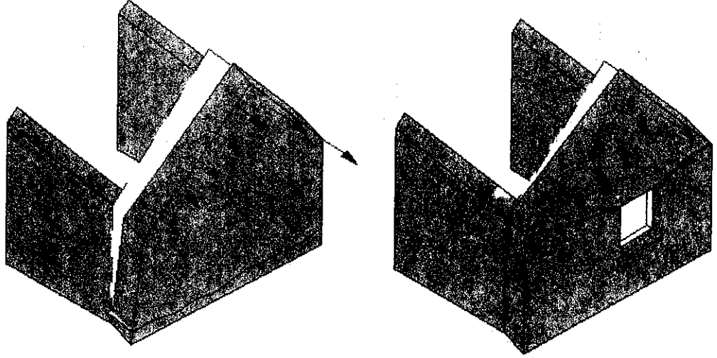
شكل 1. انقلاب وانهيار جزئي لجدار الجملون
