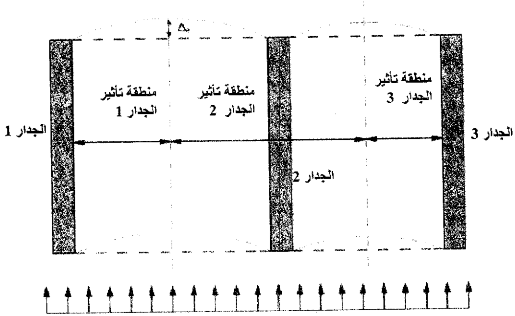
الشكل 19. أرضية تقليدية مرنة : منطقة التأثير للجدران. مكونات الزلزال في اتجاه الجدران 1، 2 و 3.
