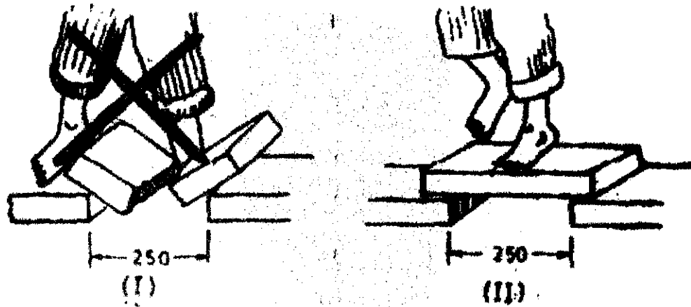
الشكل 14. تجربة كفيية لمقاومة وحدات الطوب الطيني
