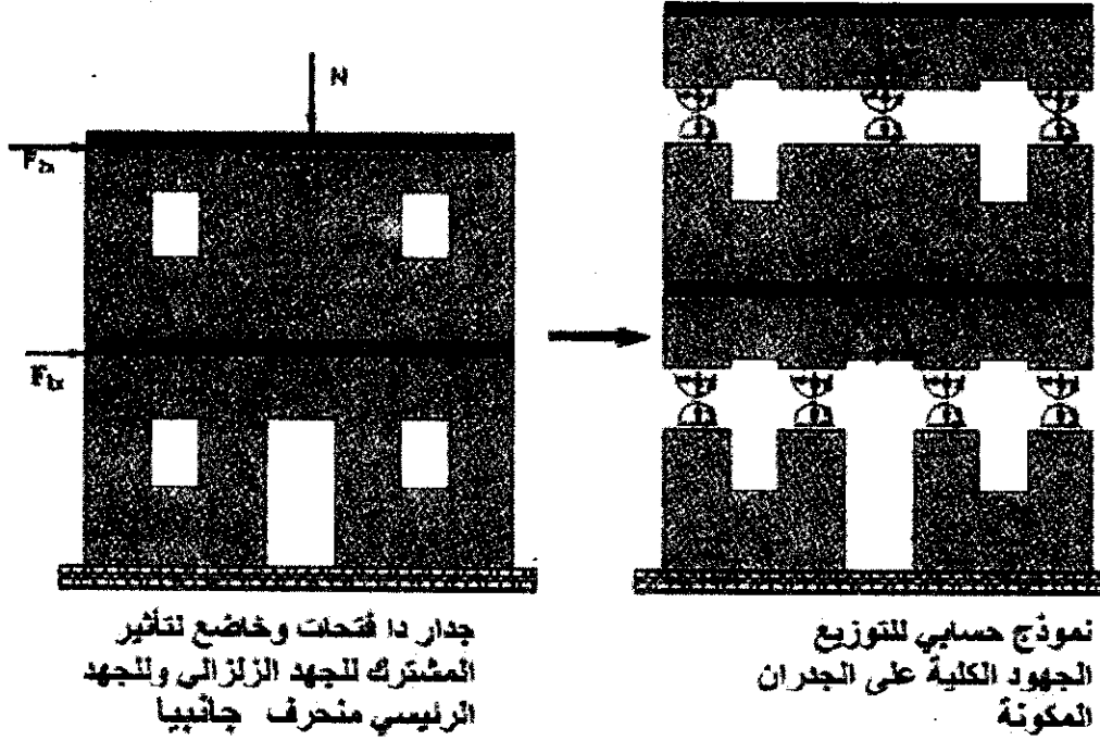
الشكل 21. نموذج توزيع الجهود الزلزالية
