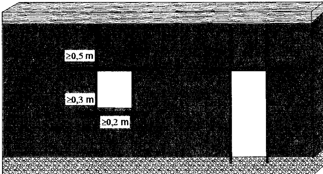
الشكل 46. تدعيم الفتحات بالموترات العمودية والأفقية
