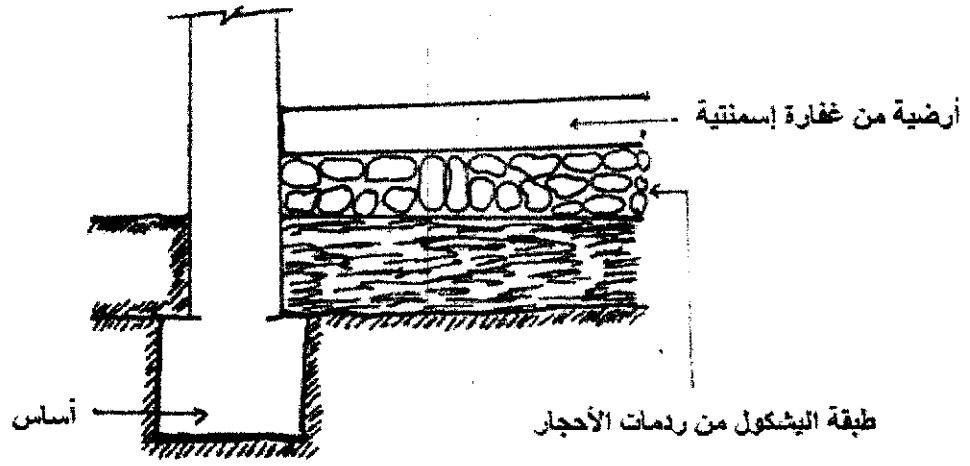
الشكل 30. تفصيل بنائي لترصيف بالموااد المحلية
