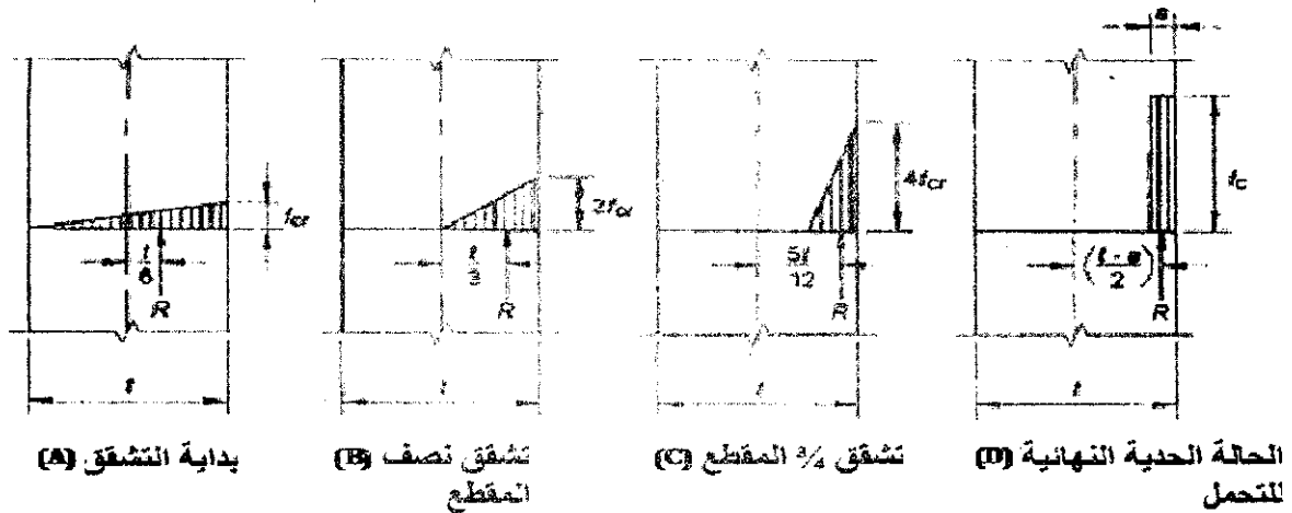
الشكل 29. توزيع إجهادات المضاغطة لمختلف حالات التشوه
