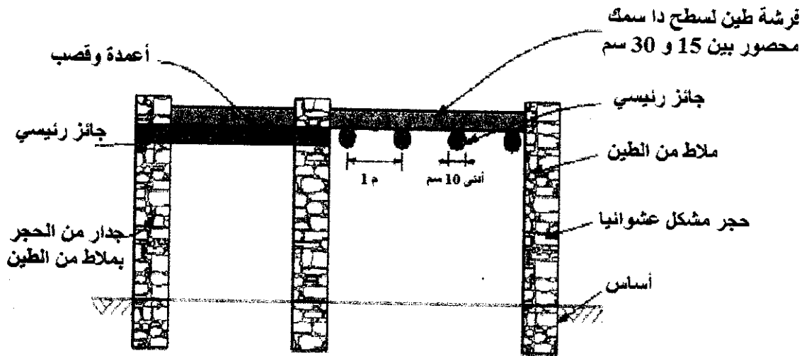
الشكل.11. رفع لبنانية تقليدية بالحجر
